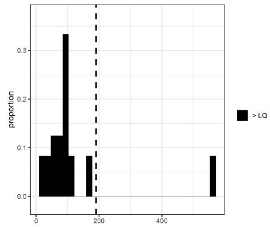
1,2,3,4,6,7,8,9-Octachlorodibenzo-p-dioxine Histogramme dégroupé LQ discretisées
