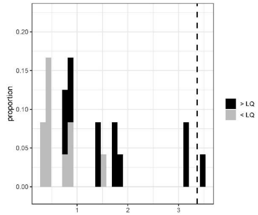
1,2,3,6,7,8-Hexachlorodibenzofurane Histogramme dégroupé LQ discretisées
