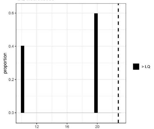
C12-C16-Coupes hydrocarbures Histogramme dégroupé LQ discretisées
