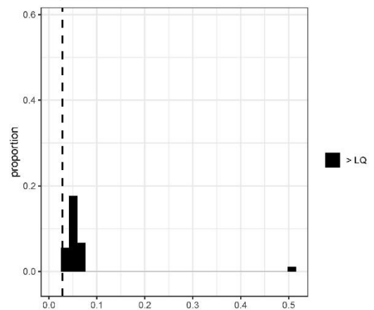
Dibenzo(a) Histogramme dégroupé LQ discretisées
