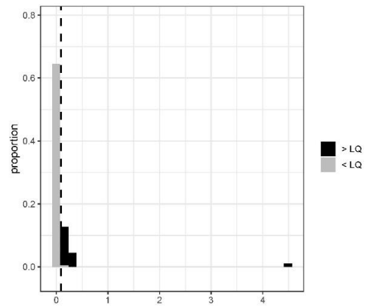
Indéno(1) Histogramme dégroupé LQ discretisées
