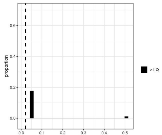
Naphtalène Histogramme dégroupé LQ discretisées
