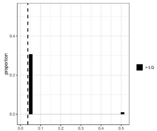
Fluorène Histogramme dégroupé LQ discretisées
