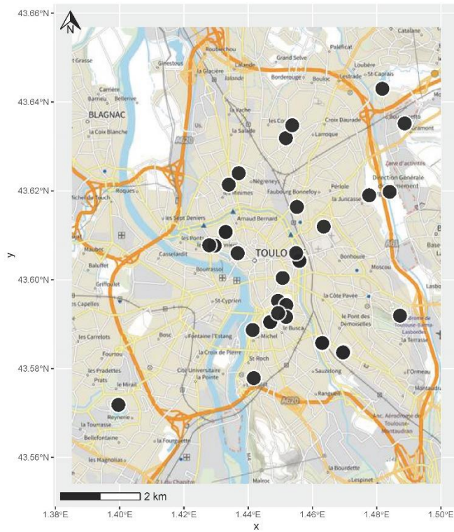
Somme 16 HAP US EPA
