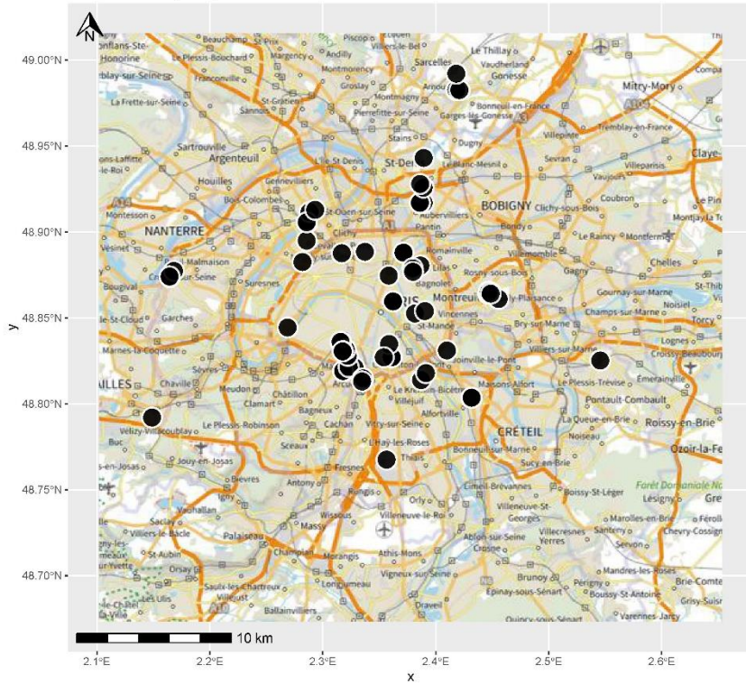
C10-C40-Coupes hydrocarbures
