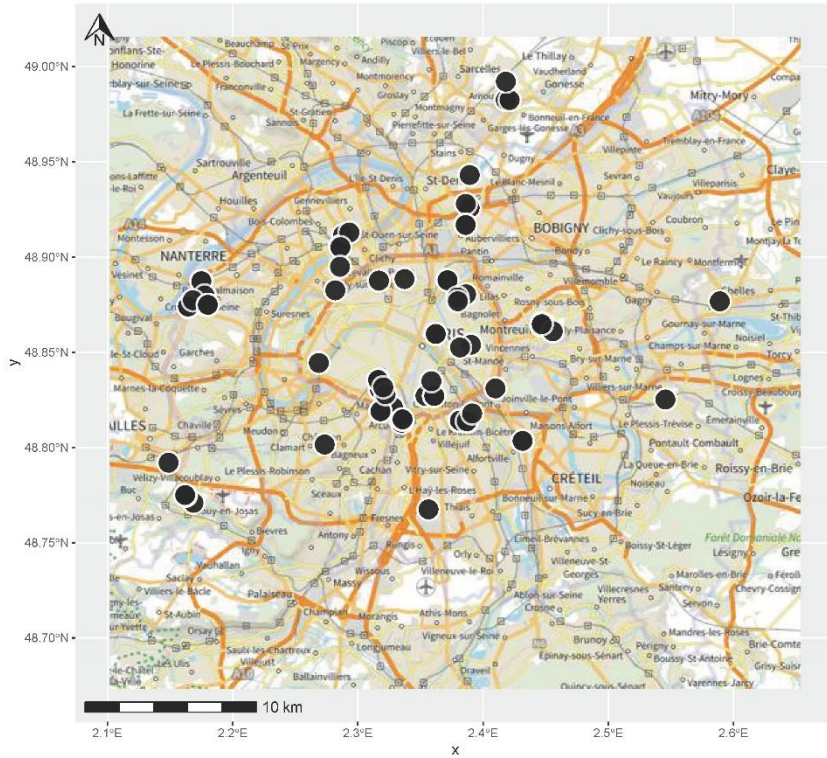
Somme 7 PCBi
